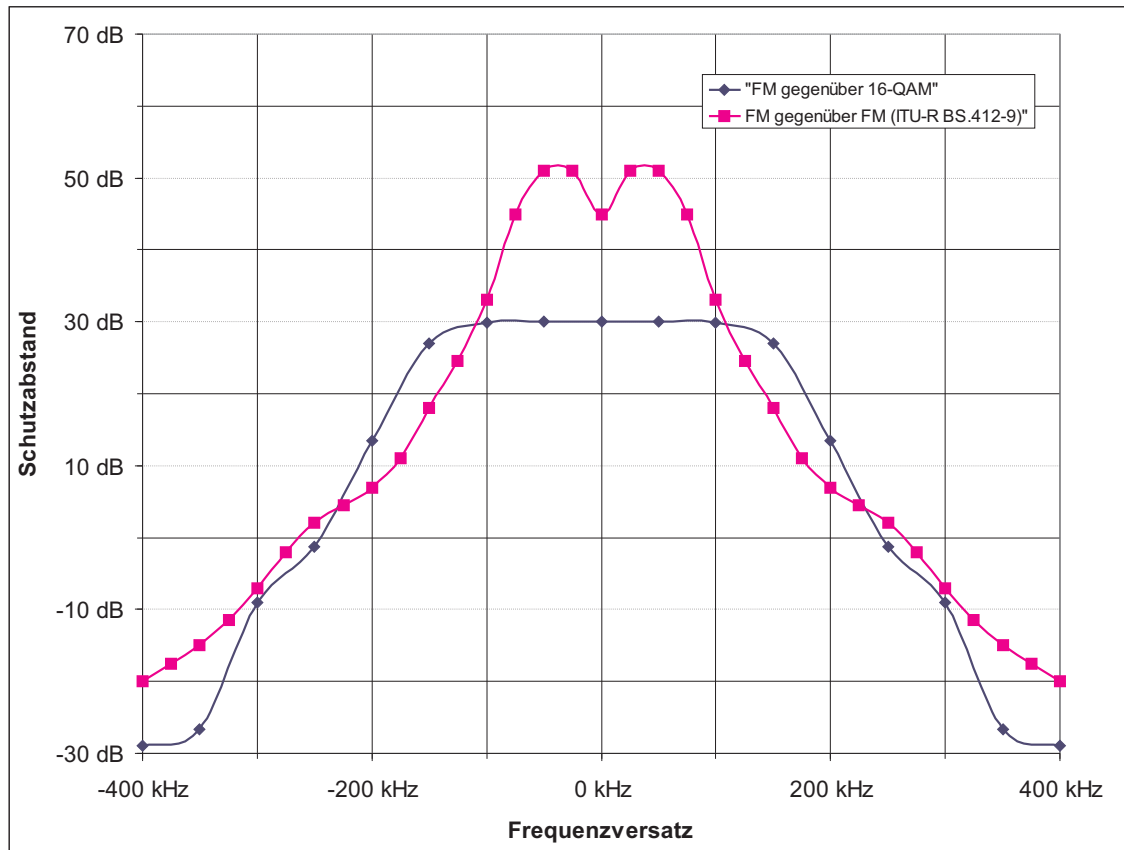
Abbildung 5.1: Schutzabstand FM gegenüber FM / DRM+
