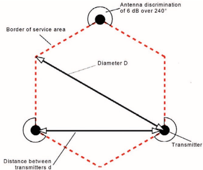
Abbildung 2.10: Geschlossenes Gleichwellennetz mit drei Sendern [8]
