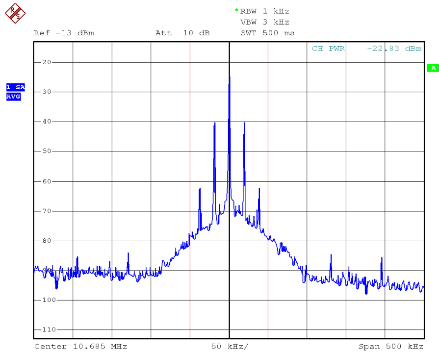
Abbildung 5.12: Erste ZF eines Empfängers - DRM+ stört FM
