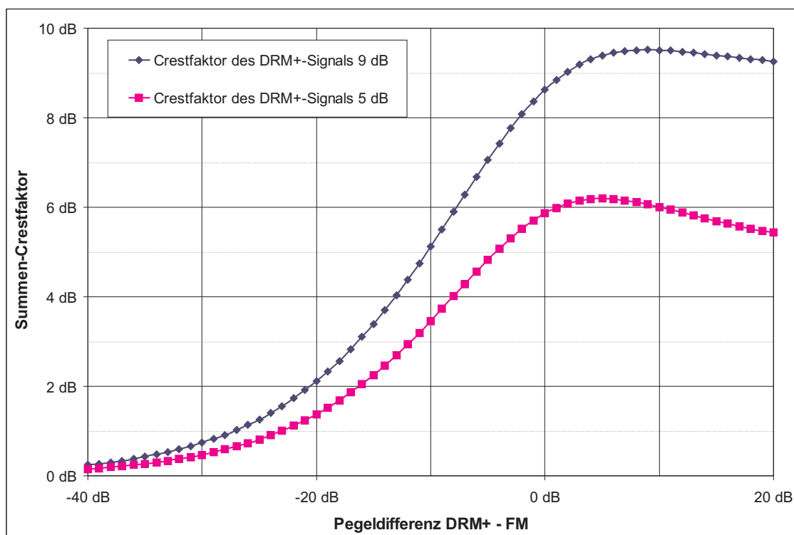
Abbildung 6.4: Summen-Crestfaktor abhängig von der Leistungsdifferenz
