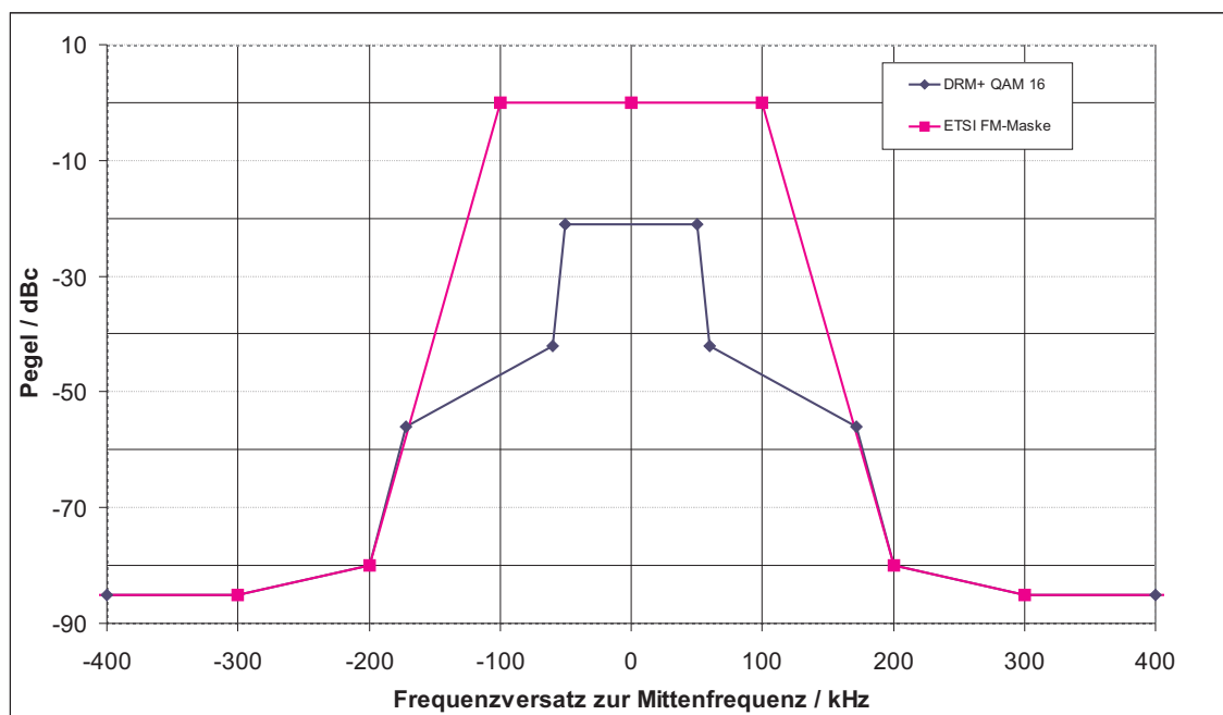
Abbildung 4.5: Sendermaske für DRM+ und FM im Vergleich
