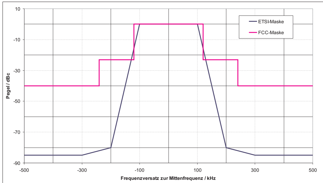
Abbildung 4.2: Spektrumsmasken für FM-Sender
