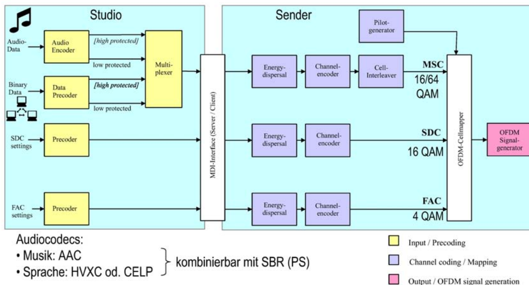
Abbildung 4.7: Aufbau eines DRM+-Signalgenerators
