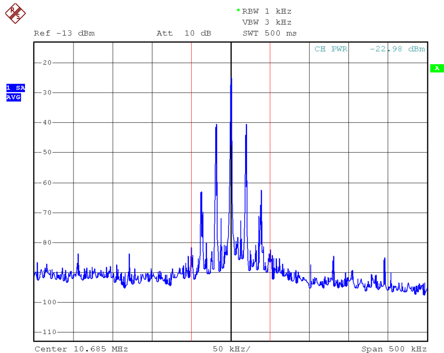
Abbildung 5.13: Erste ZF eines Empfängers - MCCW (2dB Crestfaktor) stört FM
