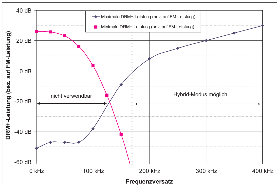
Abbildung 6.3: Minimale und Maximale Leistung eines DRM+-Signals in Abhängigkeit vom Frequenzversatz
