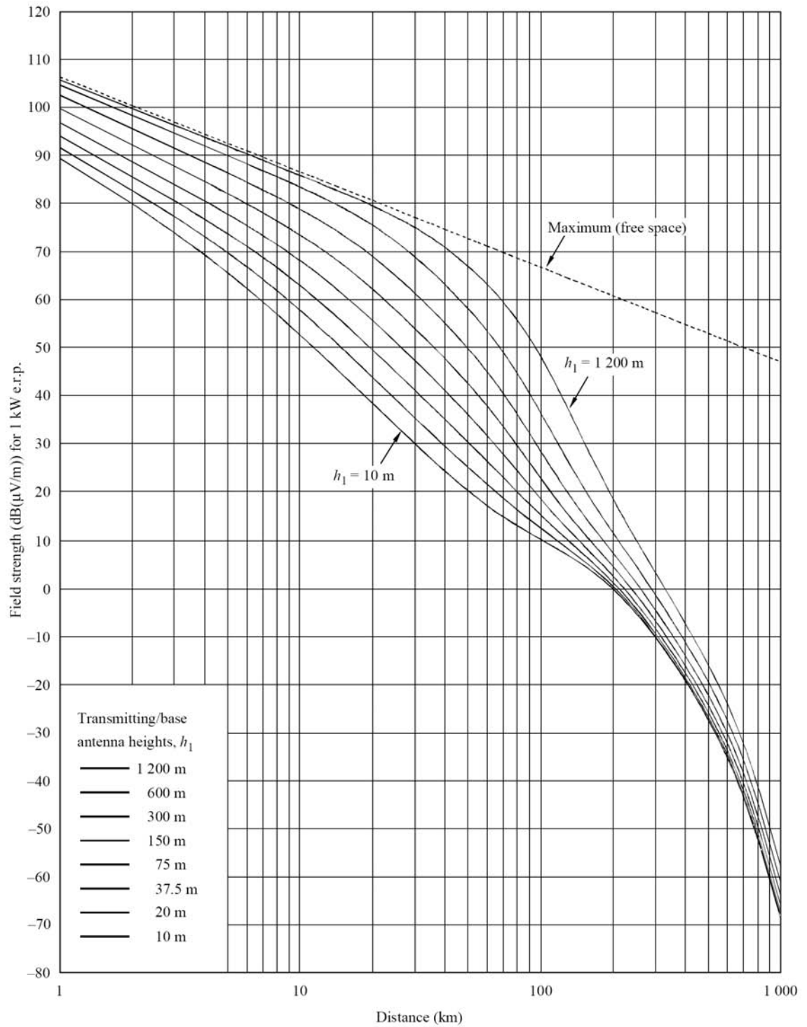
Abbildung 2.6: Ausbreitung bei 100 MHz und 50 % Zeitwahrscheinlichkeit [20]
