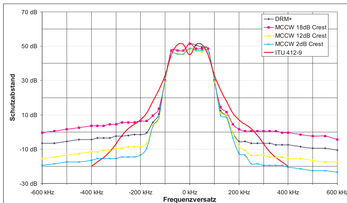
Abbildung 5.11: Schutzabstand FM gegenüber Signalen mit verschiedenen Crestfaktoren
