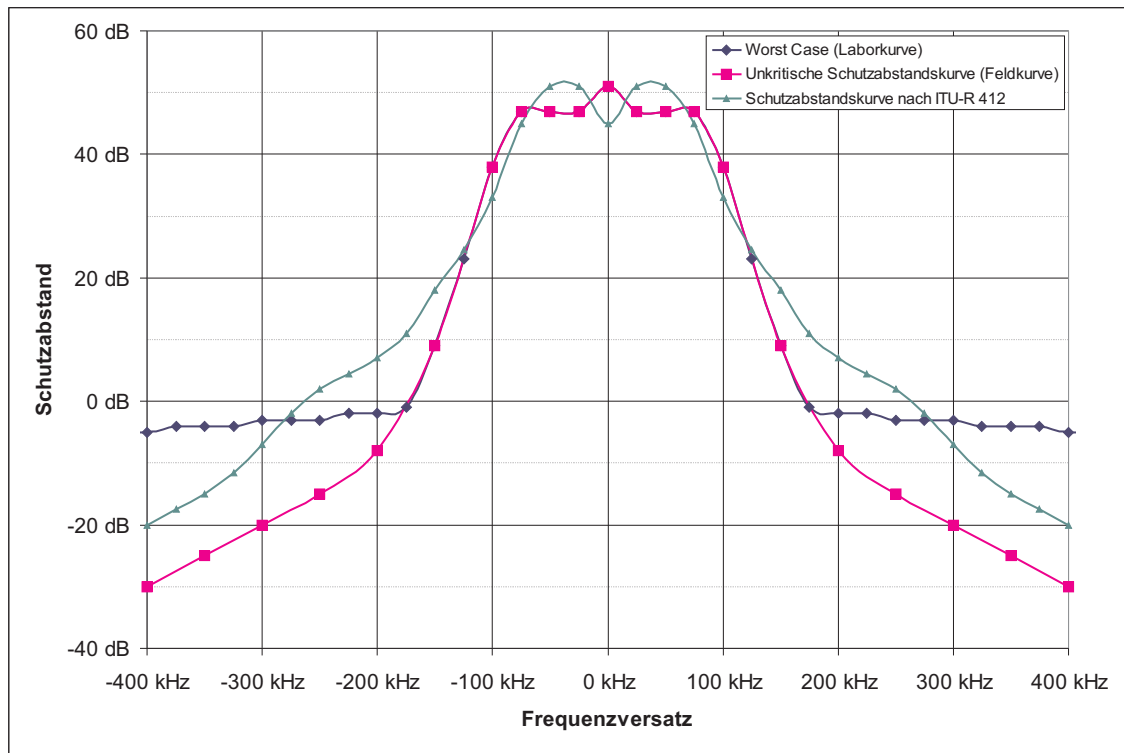
Abbildung 6.2: Kritische und unkritische Schutzabstandskurve für DRM+
