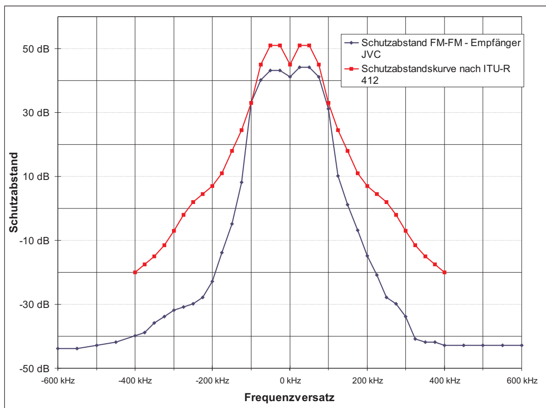
Abbildung 5.3: Schutzabstand FM-FM - Empfänger JVC
